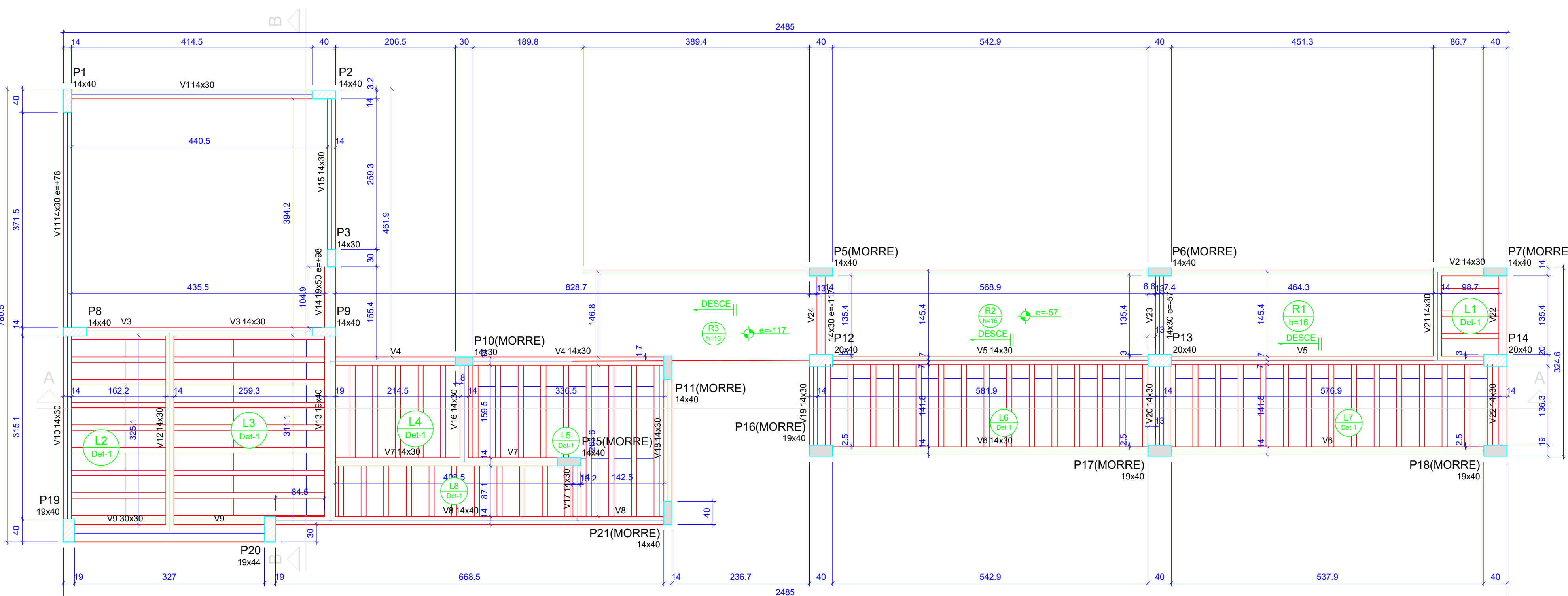
Forma do pavimento TERREO (Nível 167) escala 1:50
