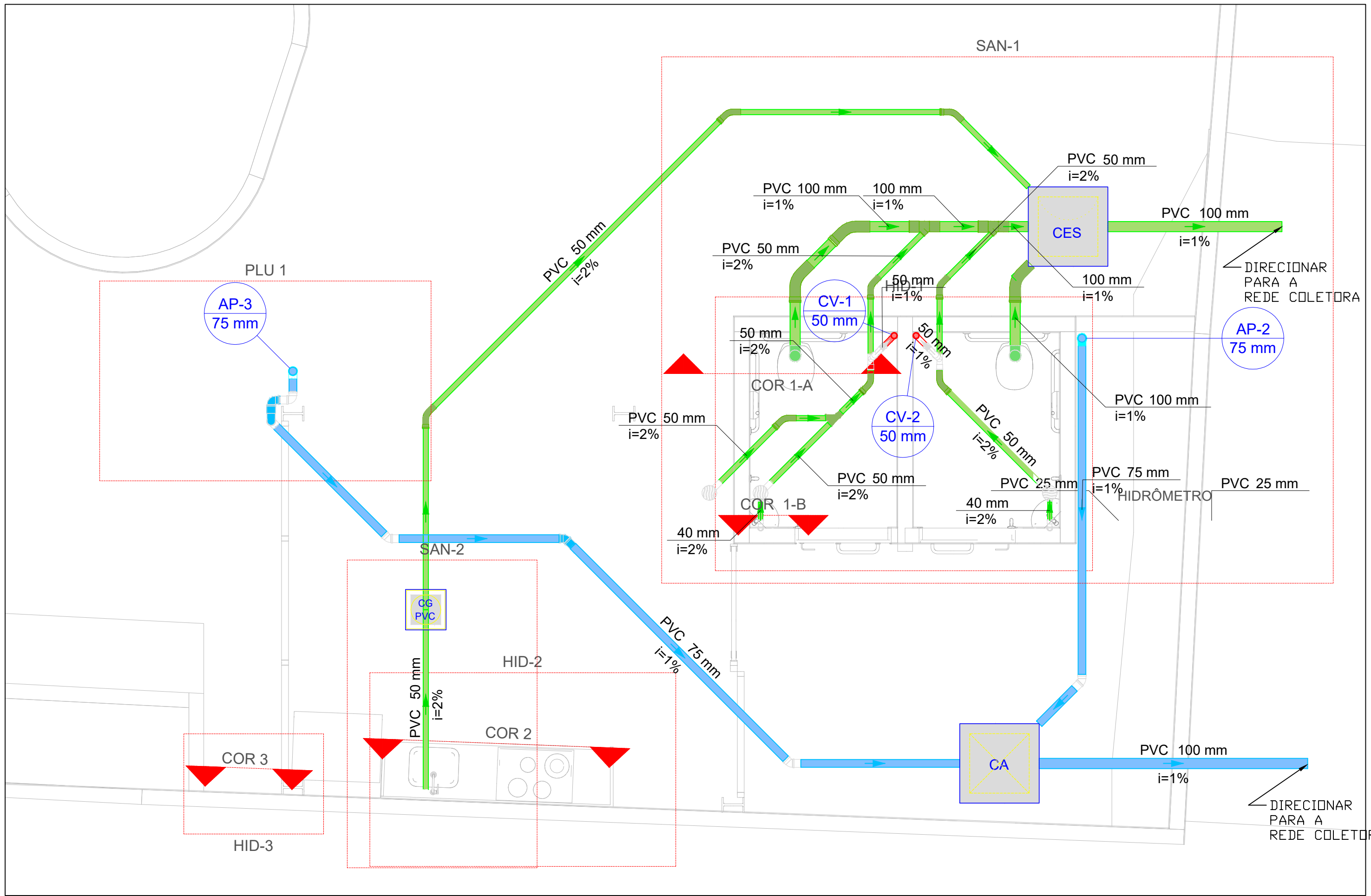
PLANTA BAIXA INSTALAÇÕES SANITÁRIAS PAV. TÉRREO ESCALA 1:50 Nível de referência : +15cm
