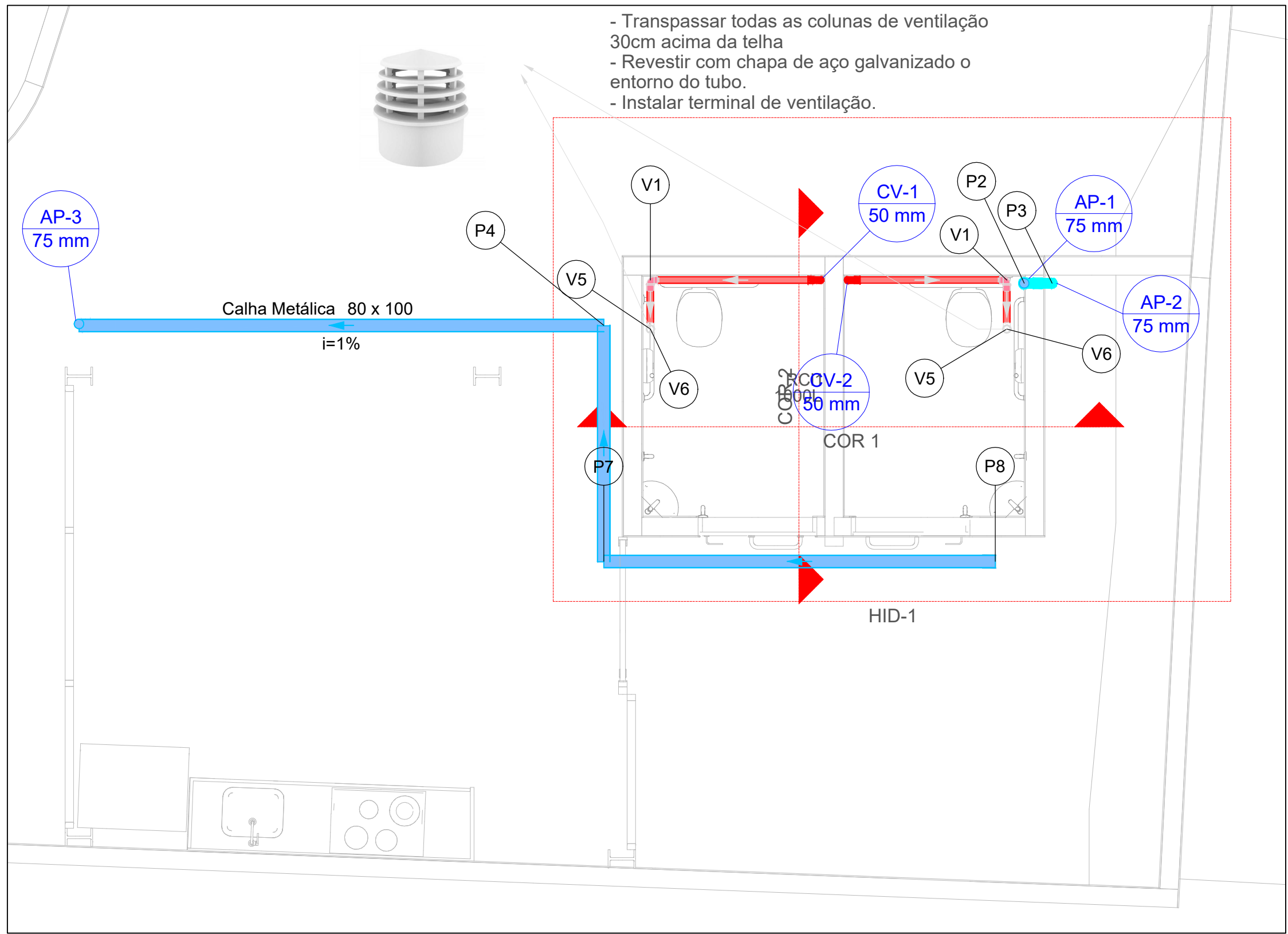
PLANTA BAIXA INSTALAÇÕES SANITÁRIAS PAV. RESERVATÓRIO ESCALA 1:50
