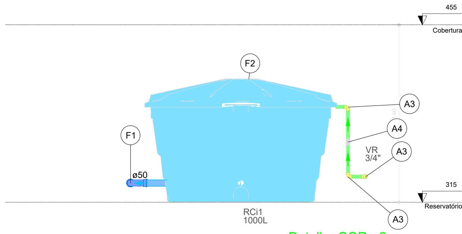
Detalhe COR - 2 Escala 1:25
