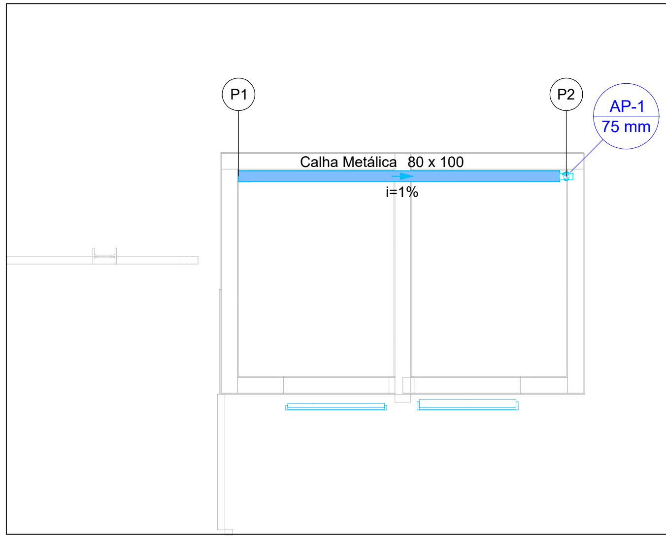
PLANTA BAIXA INSTALAÇÕES SANITÁRIAS PAV. COBERTURA ESCALA 1:50
