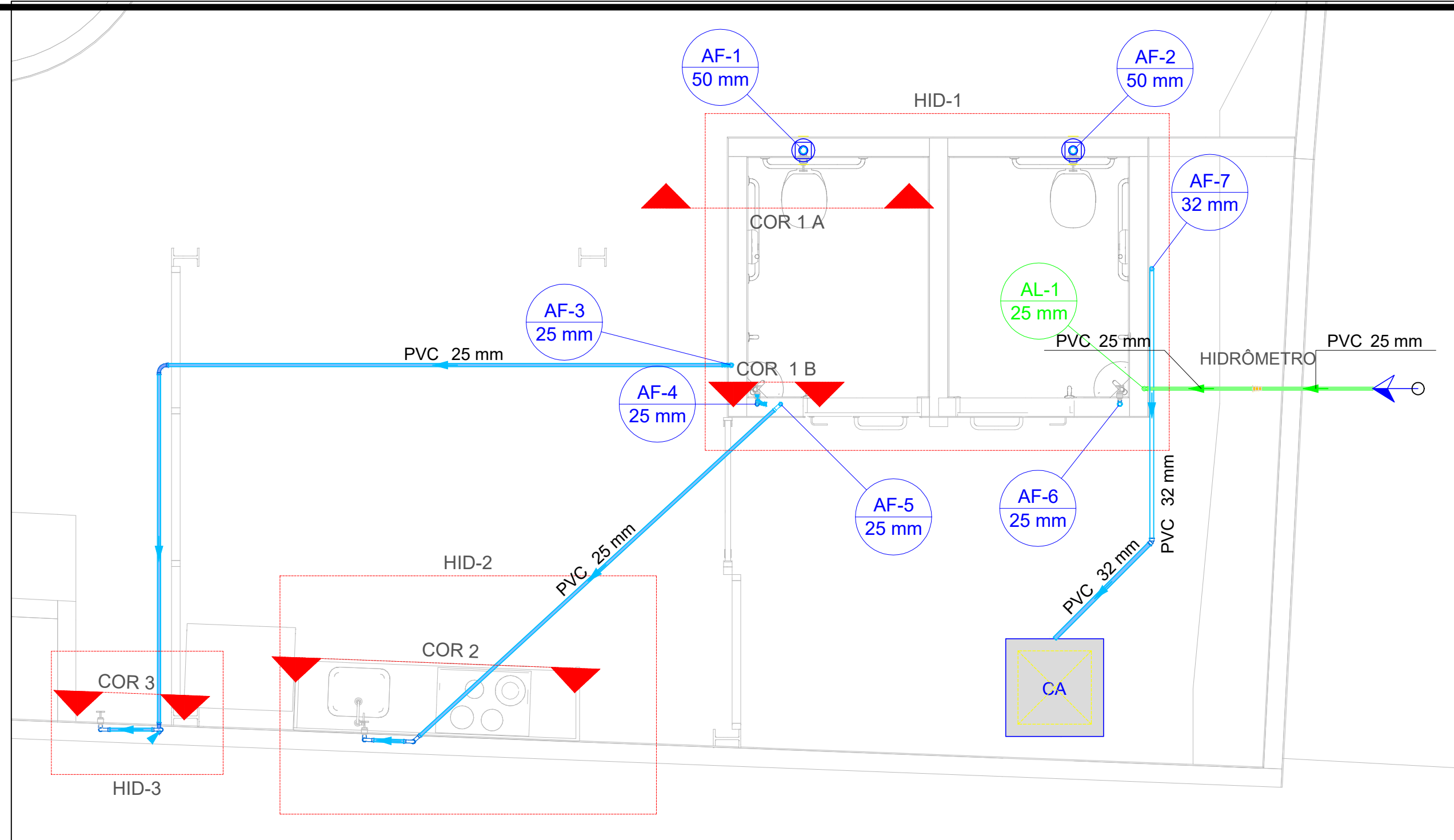
PLANTA BAIXA INSTALAÇÕES HIDRÁULICAS PAV. TÉRREO ESCALA 1:50 Nível de referência : +15cm
