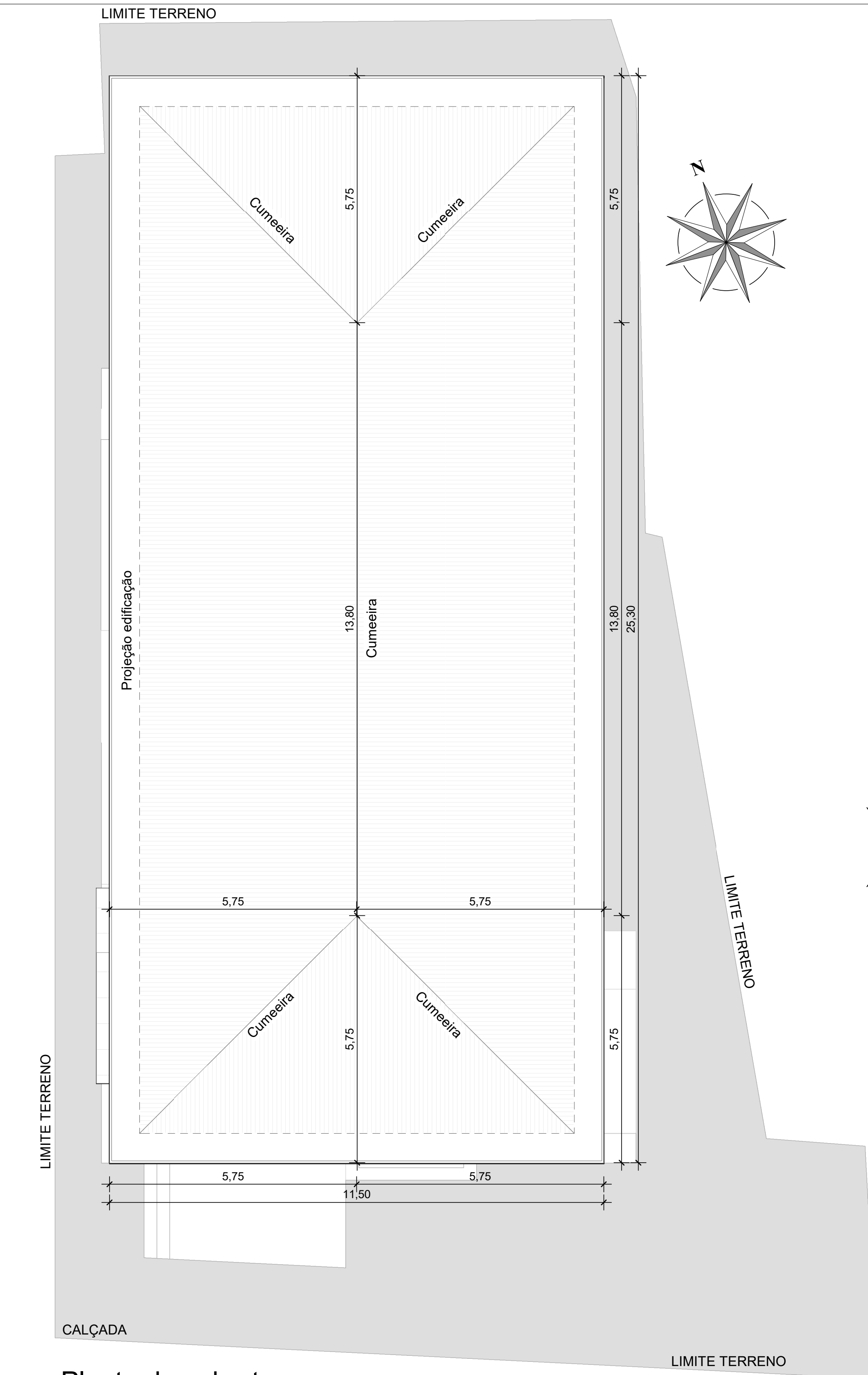
1 Planta de cobertura 1 : 75
