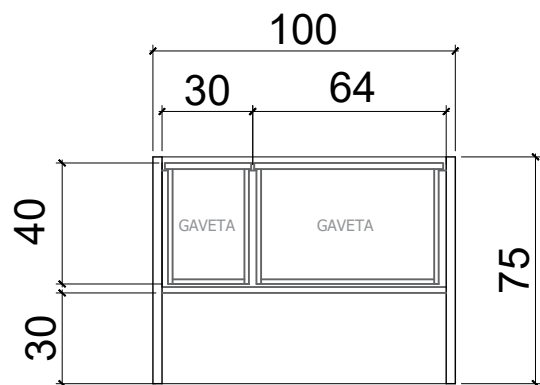
PLANTA BAIXA Cabine atendimento ESC. 1:25 INTERNO
