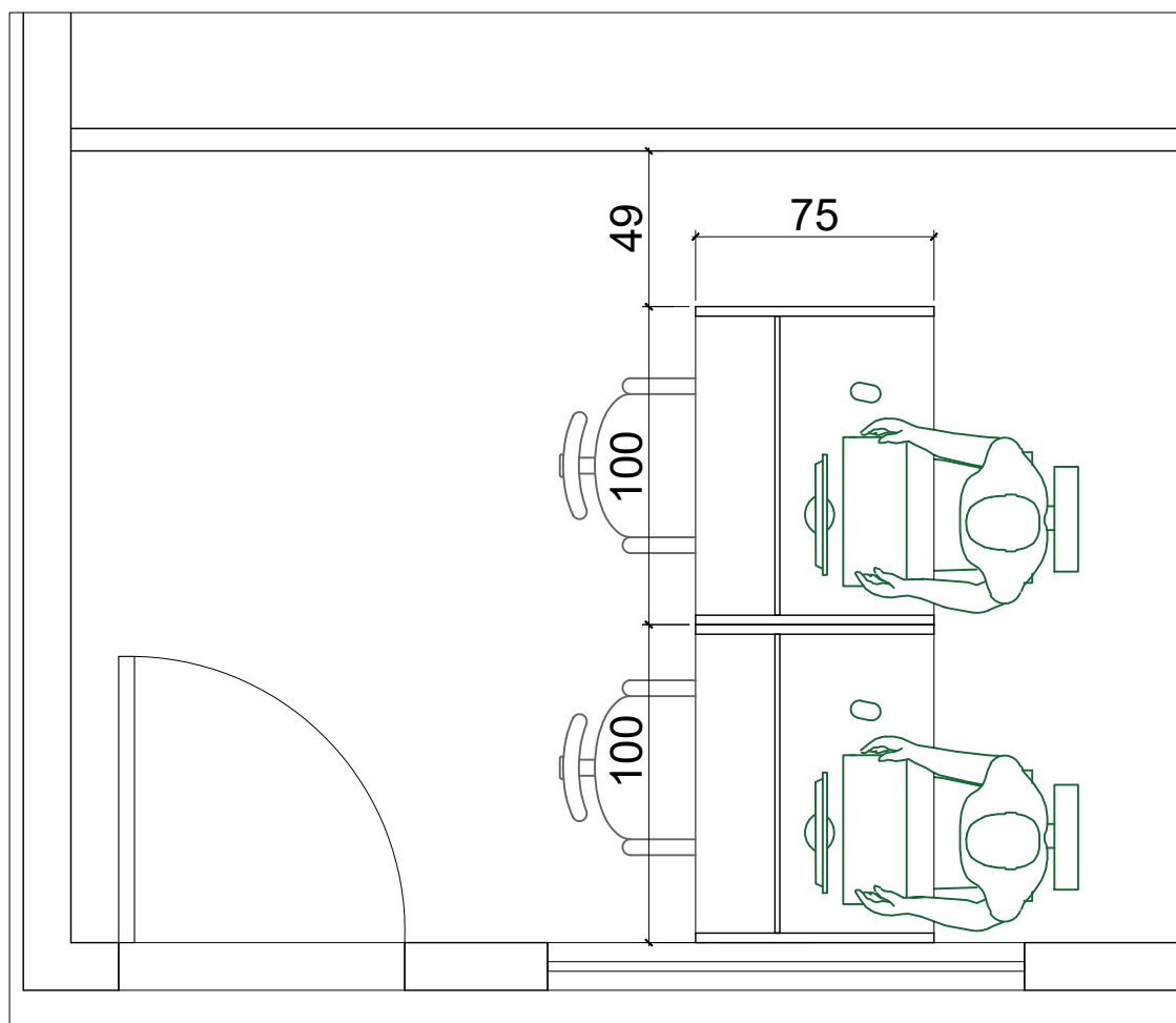
PLANTA BAIXA - Setor de SAÚDE ESC. 1:25
