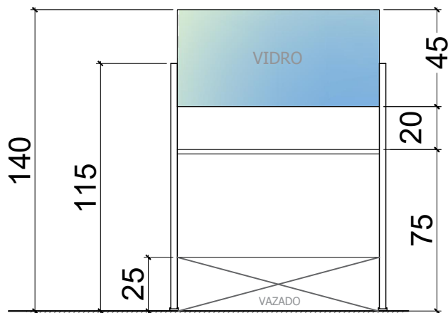
VISTA "A" - FRONTAL ESC. 1:25
