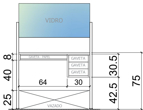
VISTA "B" - INTERNO ESC. 1:25
