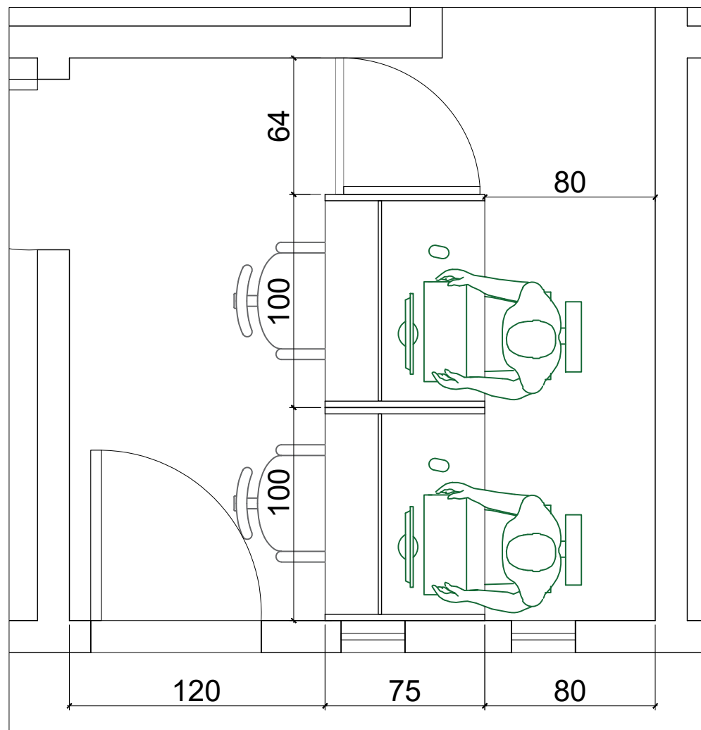
PLANTA BAIXA - Setor de R.H. ESC. 1:25
