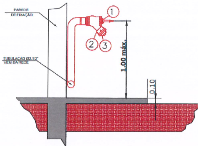
DETALHE : HIDRANTE DE RECALQUE SEM ESCALA
