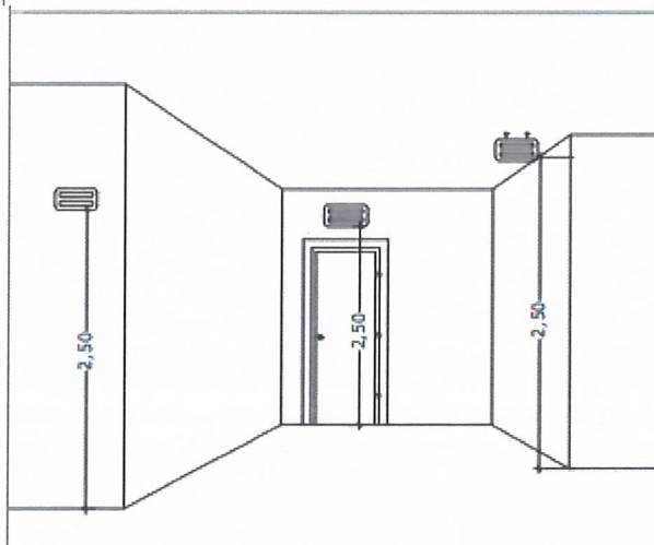
DETALHE ILUMINAÇÃO DE EMERGÊNCIA SEM ESCALA
