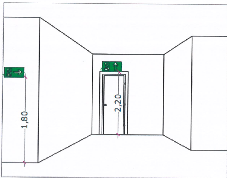
DETALHE SINALIZAÇÃO SEM ESCALA
