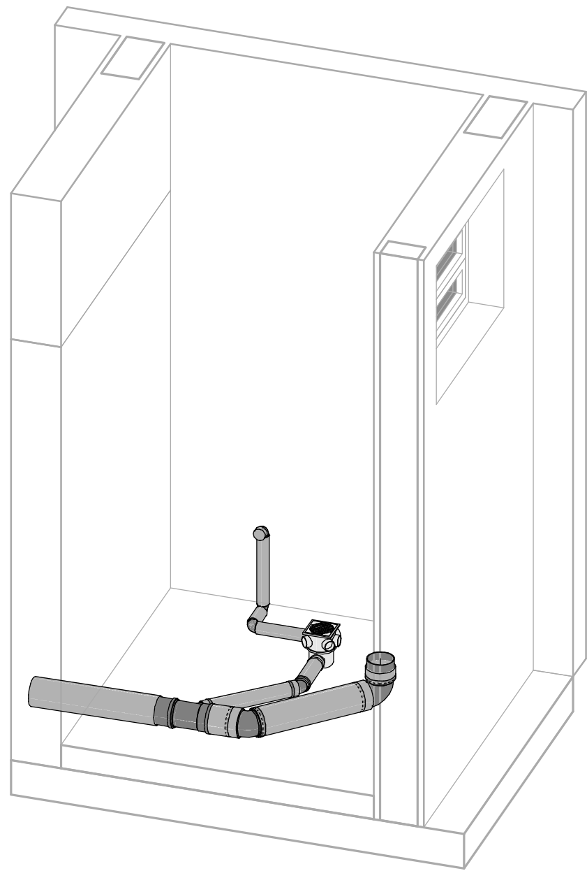
3 3D Hidrossanitário
