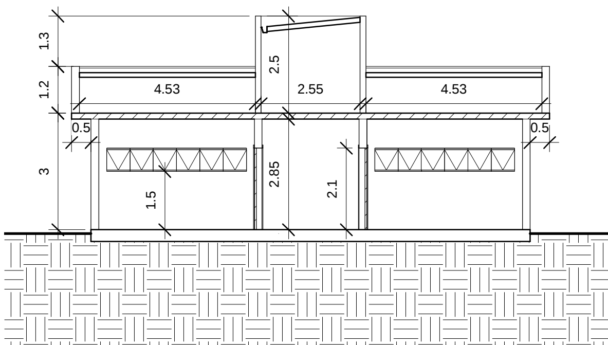
6 Corte AA 1 : 100
