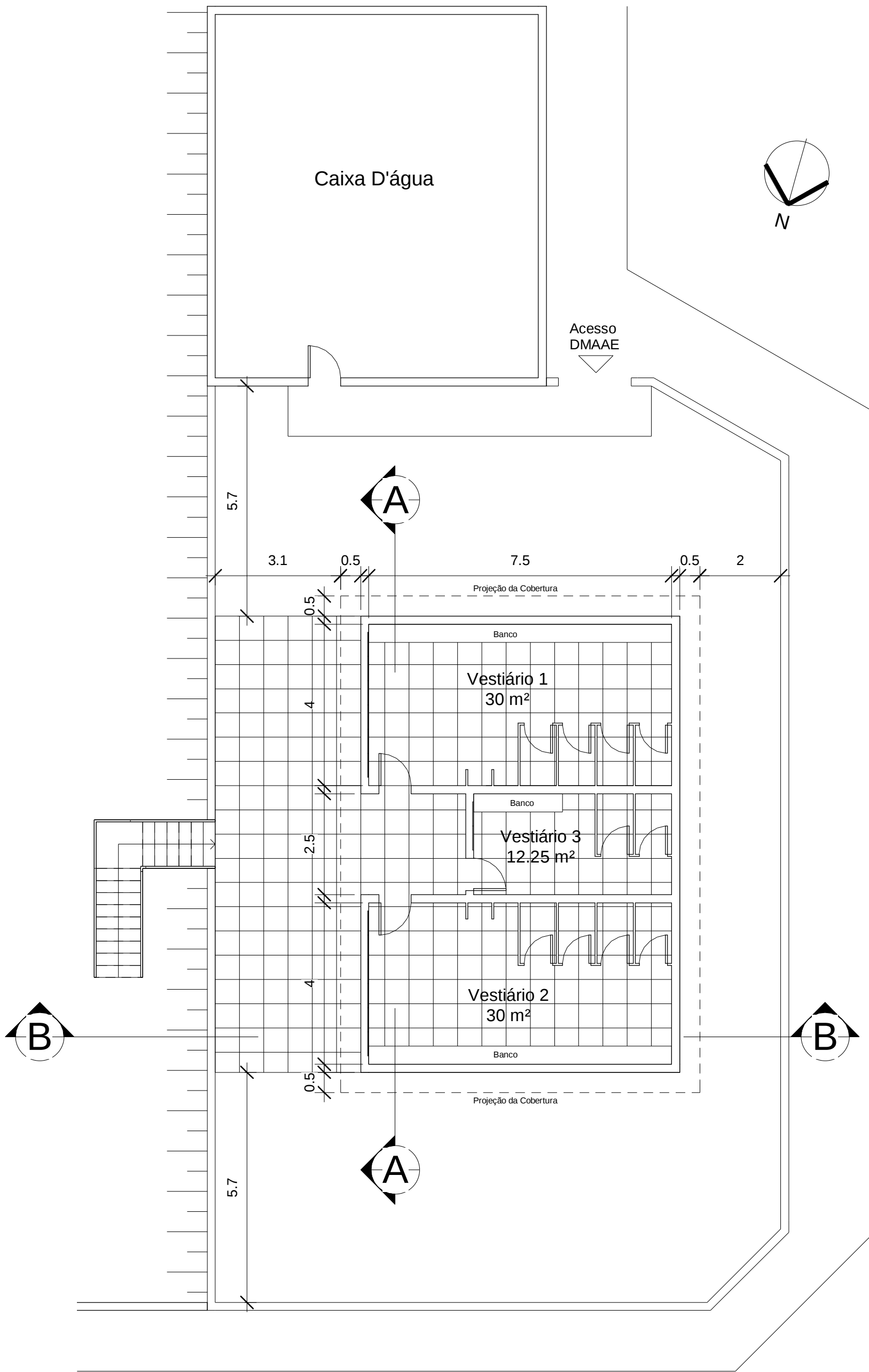
1 Planta Baixa 1 : 100
