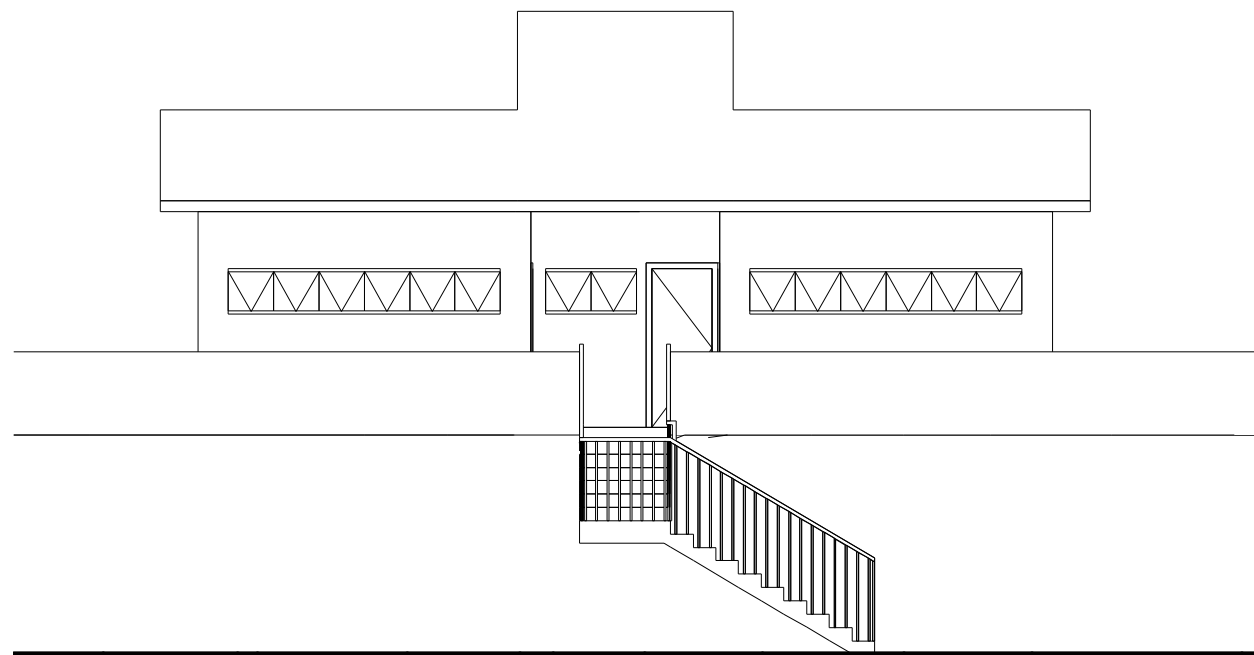
4 Vista Leste 1 : 100
