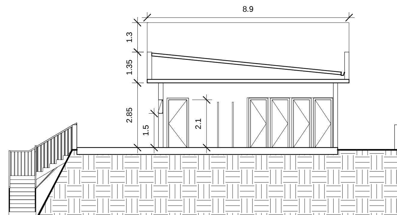
7 Corte BB 1 : 100
