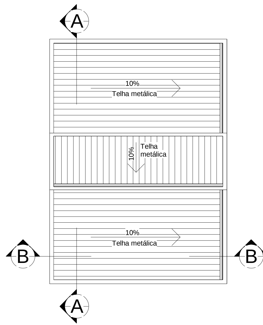
8 Cobertura 1 : 100
