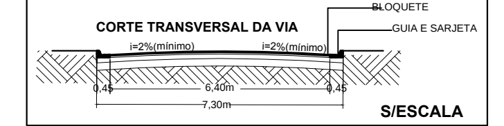
PAVIMENTAÇÃO EM BLOQUETE SEXTAVADO
