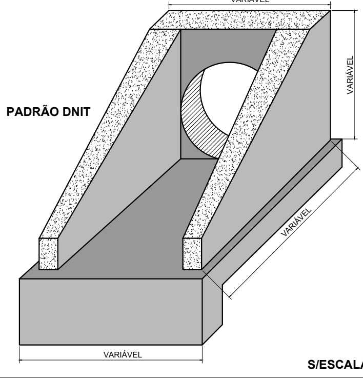
BUEIRO SIMPLES TUBULAR DE CONCRETO BOCAS NORMAIS E ESCONSAS
