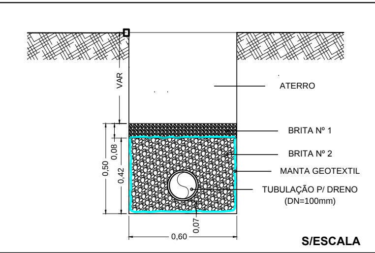
PERFIL TRANSVERSAL DA REDE / DRENO
