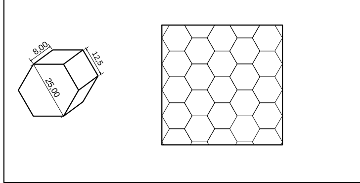
PAVIMENTAÇÃO EM BLOQUETE SEXTAVADO
